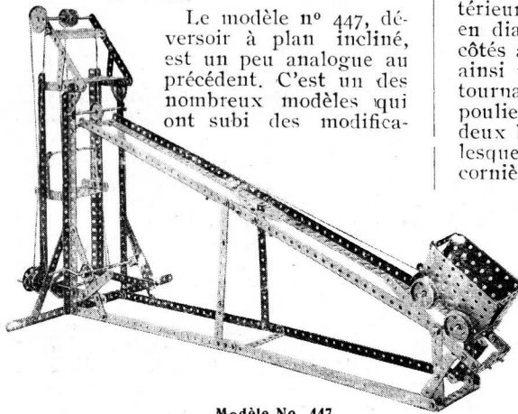
Modèle No. 447. Déversoir à Plan incliné
