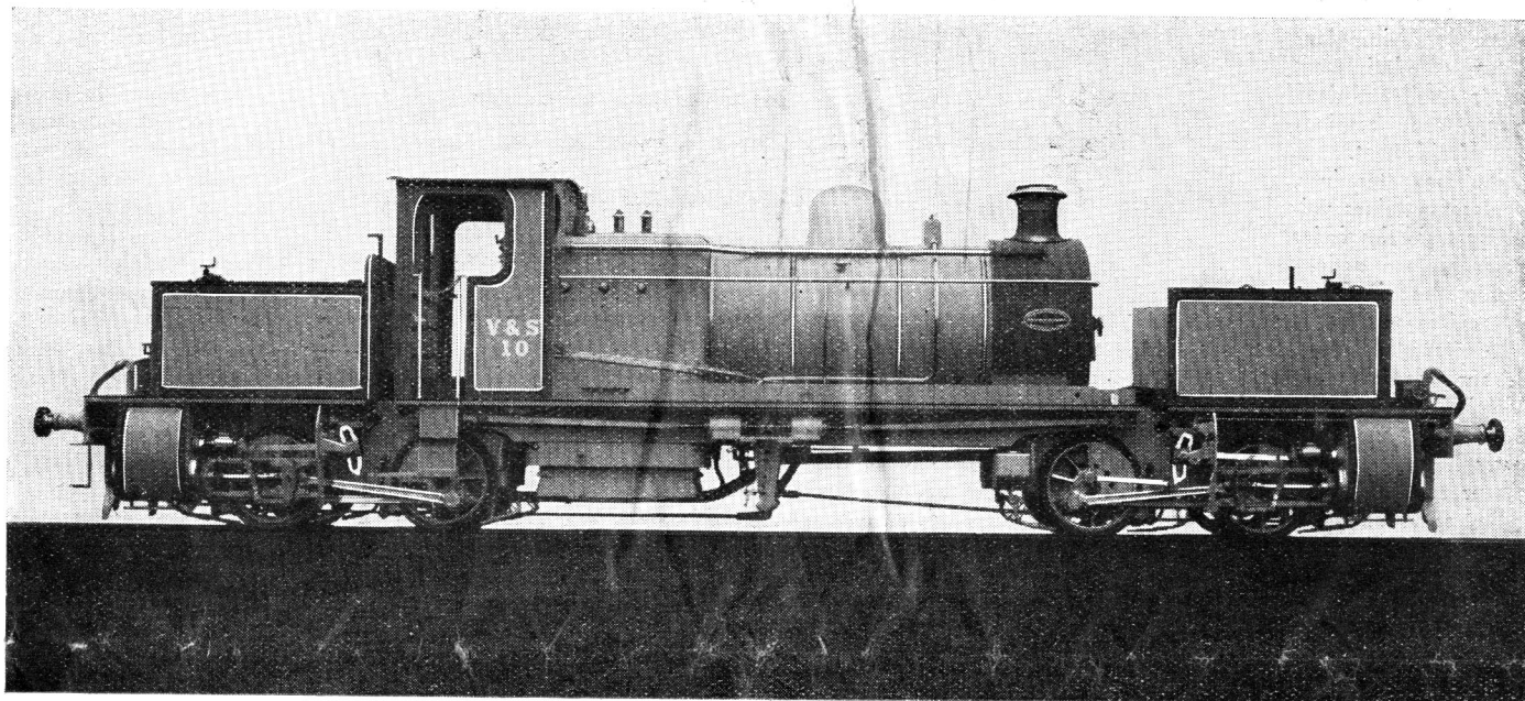
Locomotive articulée, système Garratt
