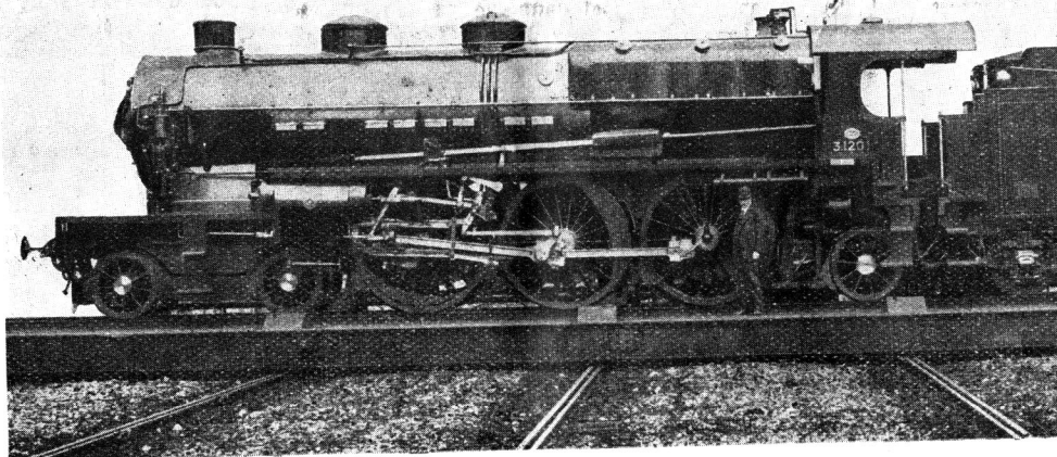
Locomotive "Pacific" de la Compagnie du Nord
