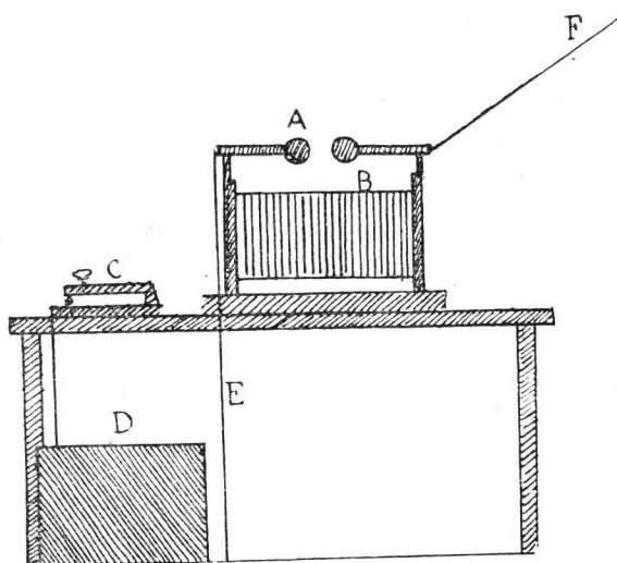
Poste Émetteur Marconi
