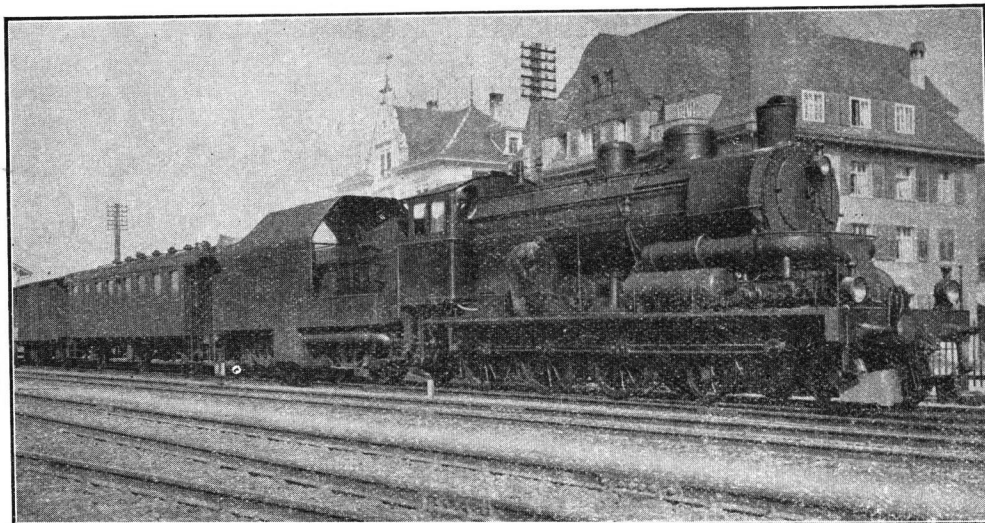
Locomotive à Turbine Système Zoelly
