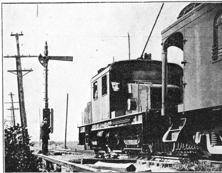
Sémaphore avec Poste Téléphonique
