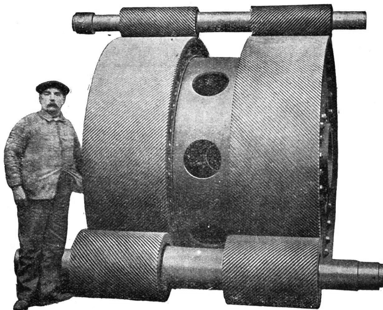
Engrenage de 23.000 H. P. pour Croiseurs
