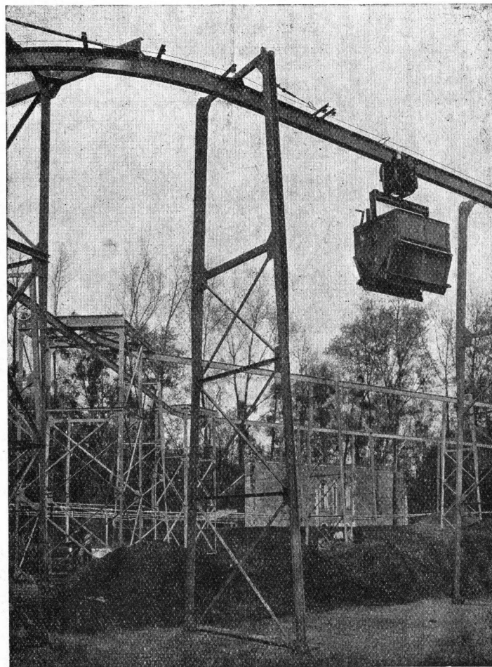
Monorail Electrique.
