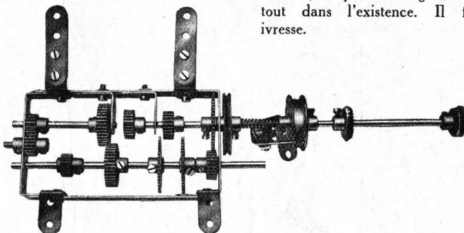
Les Boîtes d'Engrenages du Châssis-Automobile
