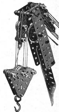
M 1. Dispositif de poulie dans le Derrick à pied rigide. (Modèle No 709)
