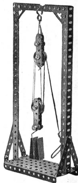
Fig. 3. Palan à deux poulies
