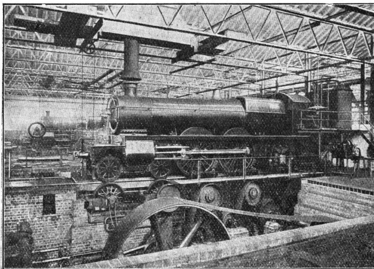
Dispositif pour l'essai "à froid" des locomotives.
