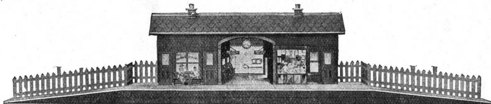
Gare Excellent modèle, d'un merveilleux dessin et d'un beau fini. Dimensions: Longueur 83 cm., largeur 15 cm., hauteur 18 cm. Prix. . . . . Frs 75 00
