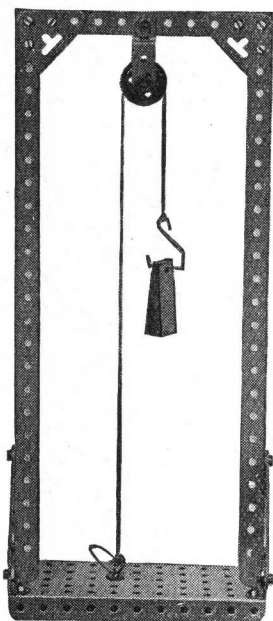
Fig. 1. Poulie fixe simple
