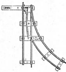
Aiguillage de gauche
