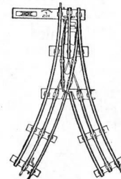
Aiguillage à double embranchements pour train électrique.
