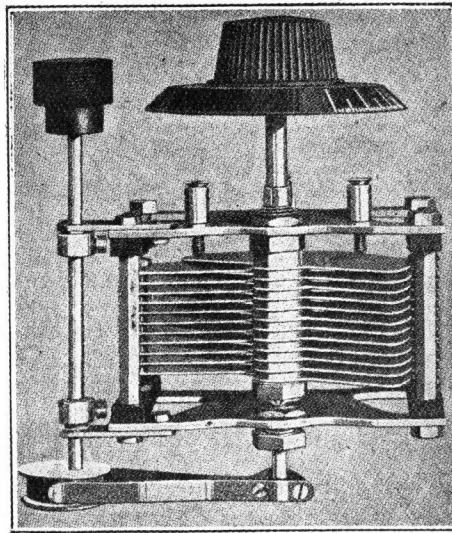
Condensateur variable. Modèle perfectionné à avance micrométrique.
