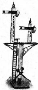
Sémaphore de Jonction Les signaux sont actionnés à l'aide de leviers.
