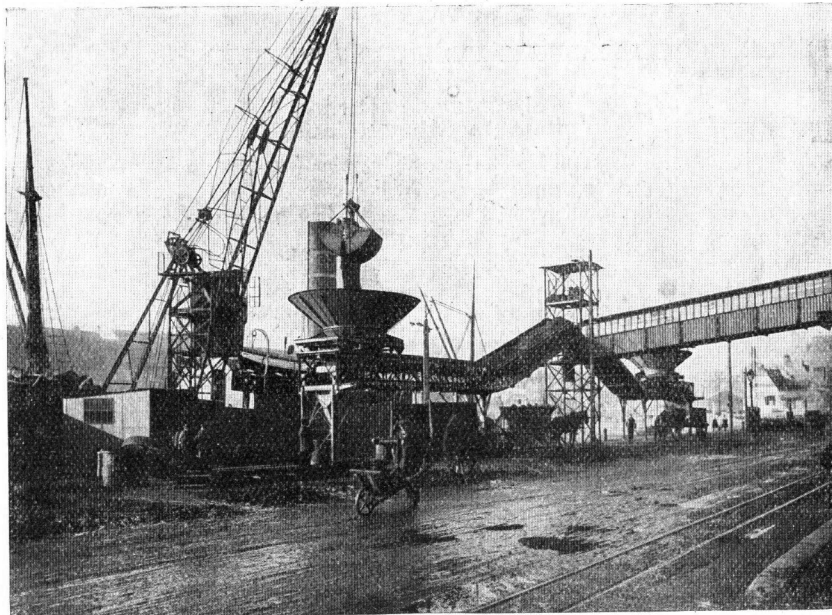
Autre aspect du Transbordeur Combiné.
