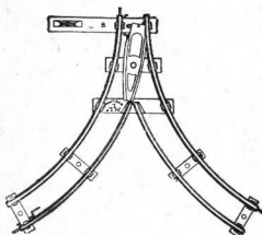
Aiguillage à double embranchements
