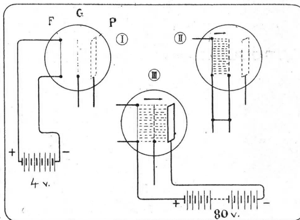
Lampe à trois Electrodes.
