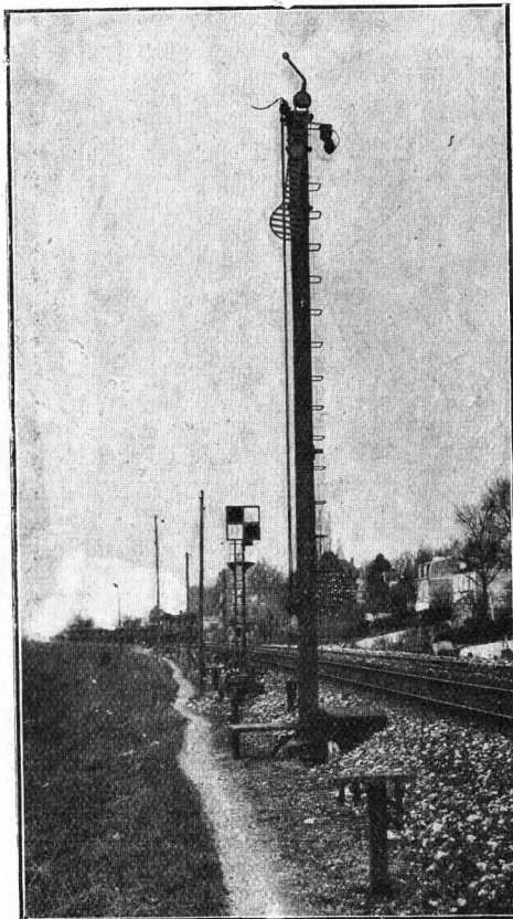
Sémaphore et Signal carré.
