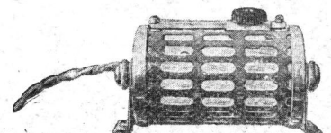
Rhéostat de réglage pour moteur 1/60
