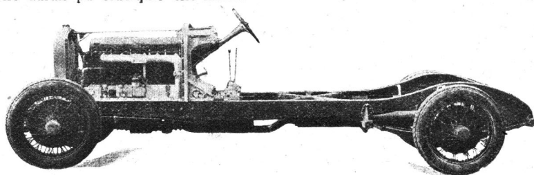
Châssis Delage.
