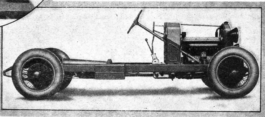
Châssis Alfa-Roméo
