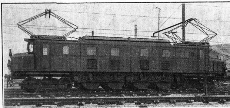
Locomotive électrique type 202 Brown-Boveri
