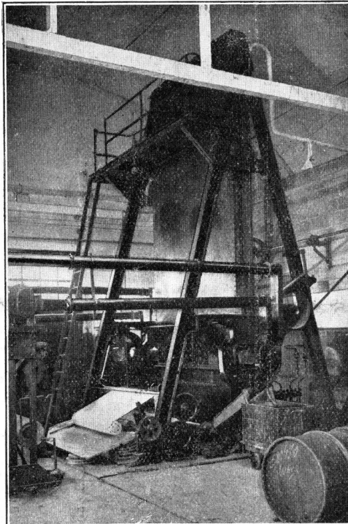
Photo) Métier à gommer vertical. (Société Dunlop
