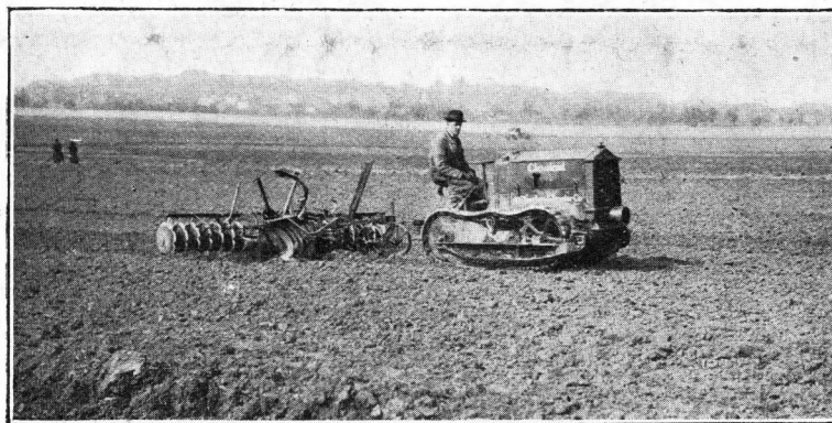
Un Tracteur « Cleveland » en travail.
