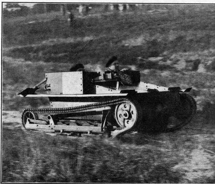
Les nouveaux Tanks anglais sont construits de façon à ne pas abimer le terrain, comme le font les Tanks ordinaires. Notre photographie représente un de ces appareils en cours d'expériences.
