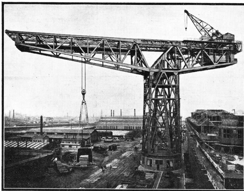
Grue Géante de 250 tonnes (Etab ts Demag)
