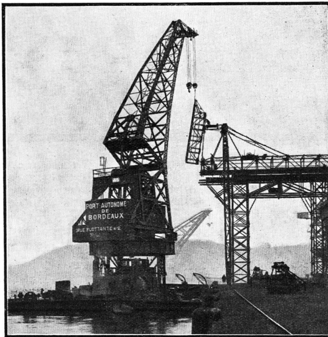
Grue flottante automotrice de 30 tonnes de puissance A l'arrière-plan, grue de 250 tonnes des Chantiers de la Gironde
