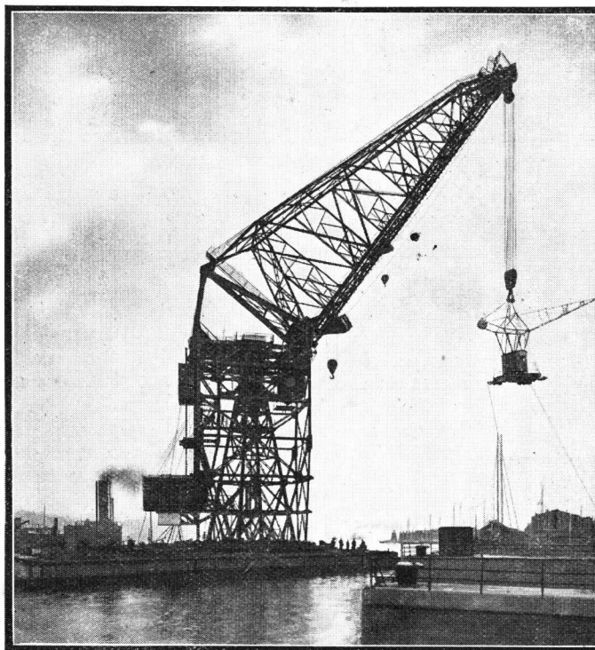
Grue Flottante de 150 tonnes (Etab ts Demag)
