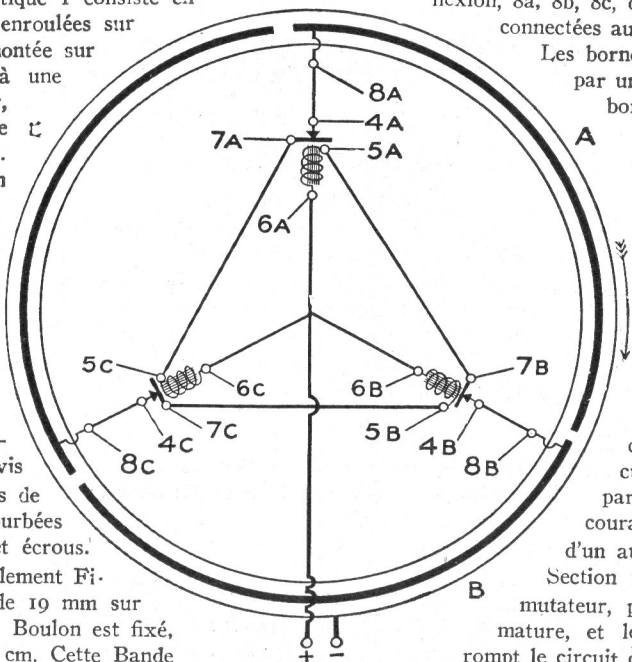
Fig. 3. — Schéma des connexions électriques.
