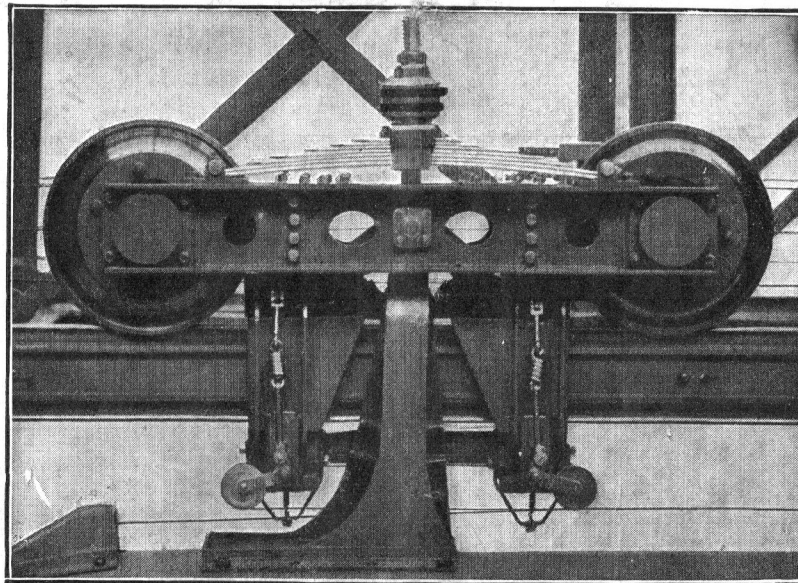
Un des bogies de suspension.
