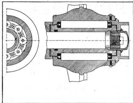
Fig. 3. Fusée d'Essieu à Rouleaux. (1856)
