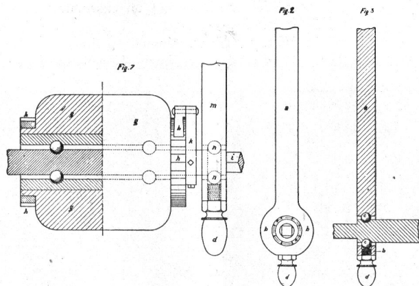
Fig. 5. Coussinet à Billes de Suriray.
