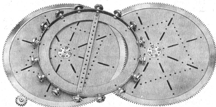
Roulement à Rouleaux Meccano.
