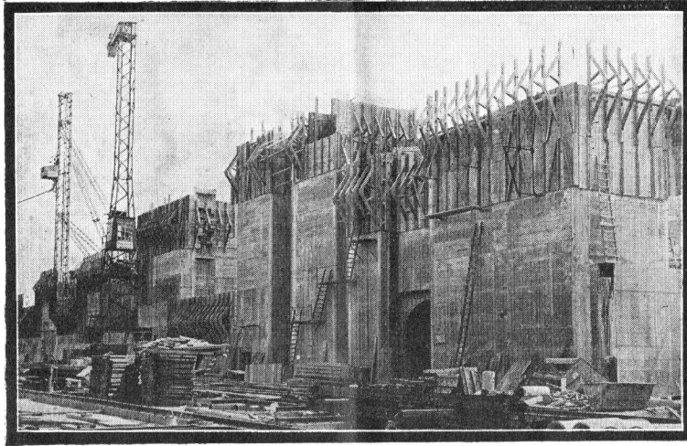
Fig. 3. L'état actuel des écluses.
