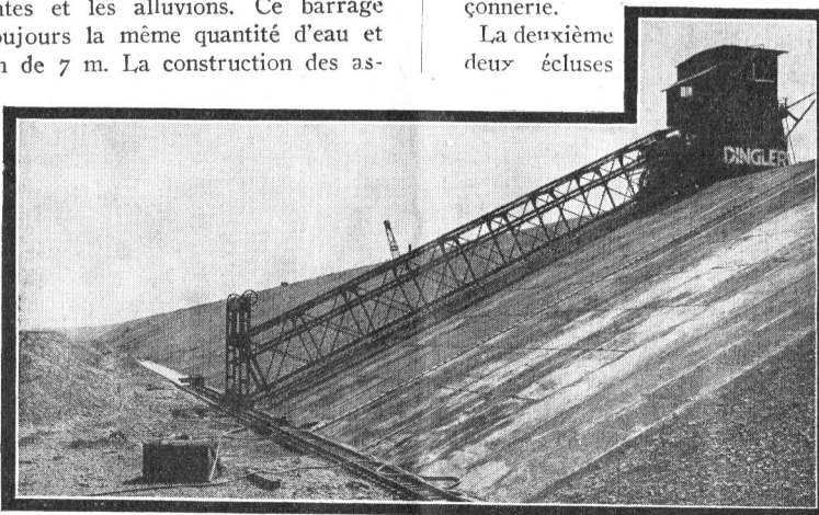
Fig. 2. Le long du canal d'aménée. — Bétonneuse Dingler.
