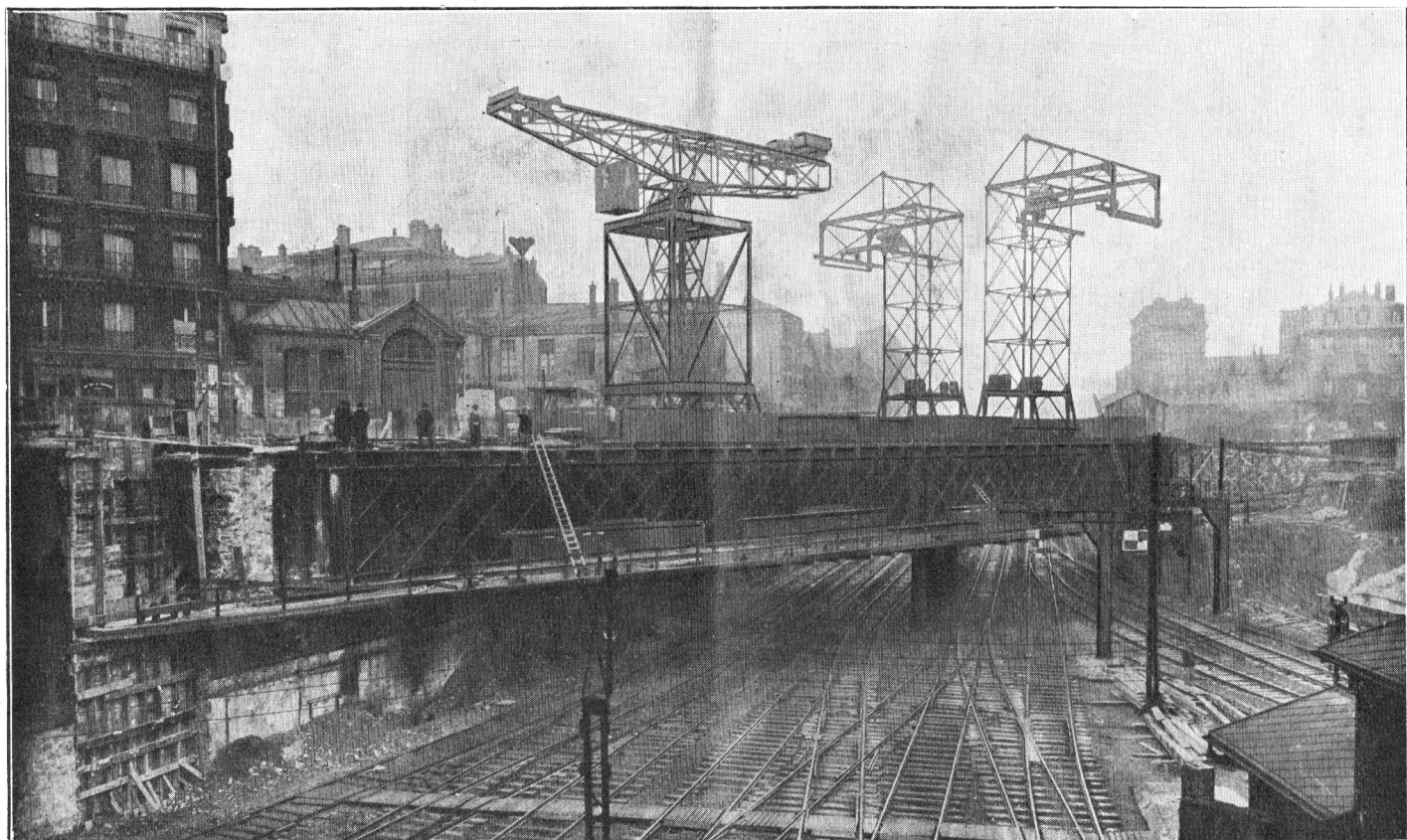
Vue du Pont de l'Aqueduc en reconstruction.
