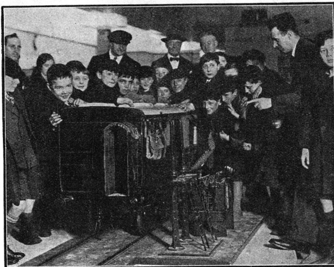
Modèle réduit du fameux « Wagon Postal Automatique », qui est en service entre Londres et Glasgow et prend automatiquement la poste à son passage sans s'arrêter. Les sacs postaux sont placés sur des filets en acier. Au passage du train, les filets basculent automatiquement et déversent leur contenu dans un autre filet accroché au wagon.
