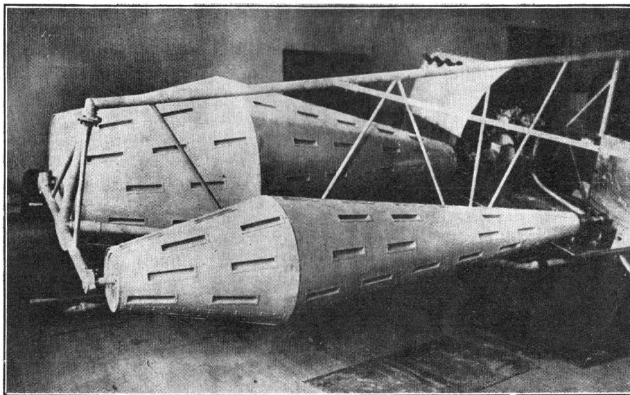
Cet original appareil, construit par deux ingénieurs américains, comporte quatre fuseaux remplaçant les ailes. Il est muni de 3 moteurs, un seul sert à la traction, les deux autres à deux cylindres doivent faire tourner les fuseaux. L'appareil pèserait 700 kgs, son envergure serait de 7 mètres et sa longueur 5 m. 50. Cliché communiqué par « l'Air ».
