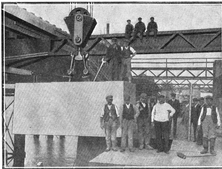
La pose du dernier bloc géant de la jetée du port de Douvres par un puissant pont roulant.
