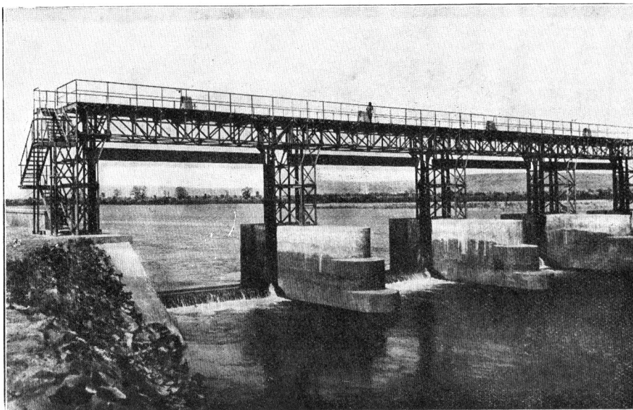
Prises d'eau du Canal de Sotuba. Passerelles des vannes (abaissées). Les clichés de cet article ont été mis à la disposition du M. M. par le « Génie Civil »
