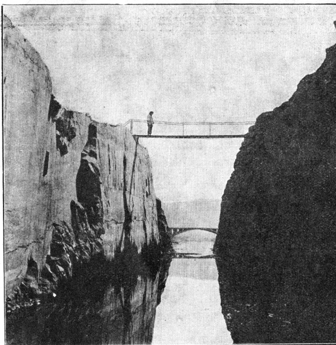
Vue du Canal de Sotuba. Traversée de l'éperon rocheux.
