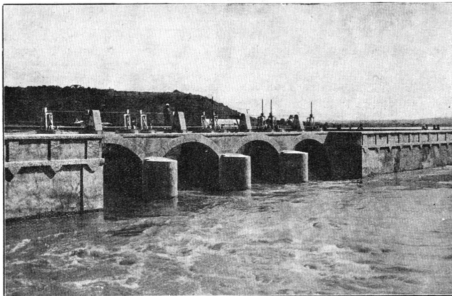
Prise d'eau du Canal de Sotuba. Ouvrage de prise d'eau. Vue prise en Amont.
