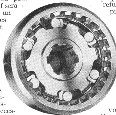
Vue intérieure du mécanisme de la roue libre Citroën.
