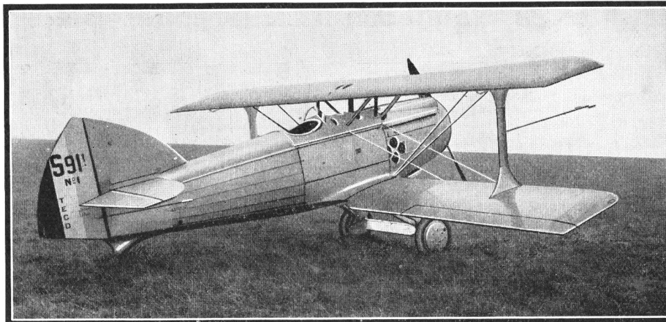
Le biplan de combat français Blériot « Spad 91-C1 ». La comparaison de cet appareil moderne avec la « Demoiselle » de Santos-Dumont (voir page ci-contre) fait valoir le progrès fait dans la construction des biplans depuis les premiers jours de l'aviation.
