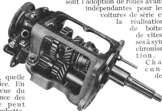
Vue intérieure de la nouvelle boîte de vitesses Citroën, montrant les engrenages silencieux et le mécanisme synchroniseur. Cette photo, ainsi que celle du mécanisme de roue libre (page ci-contre), nous a été confiée par les Etablissements Citroën.
