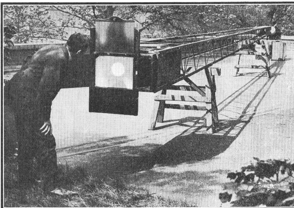
Appareil photographique géant mesurant 13 m. 50 de long. et utilisé lors d'une éclipse solaire pour photographier le Soleil. L'image du Soleil, ainsi qu'on le verra, est distinctement visible sur le verre dépoli de l'appareil.
