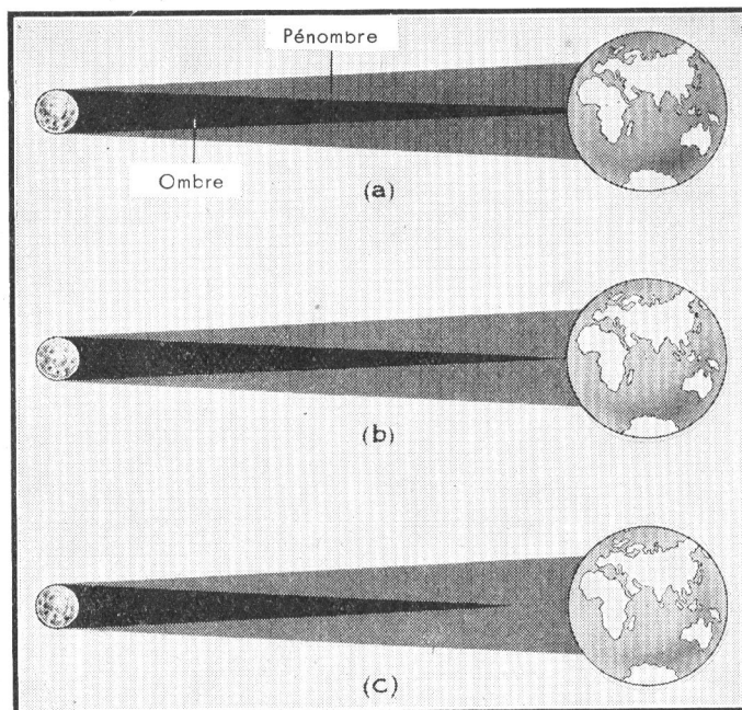
Les trois manières différentes de la répartition de l'ombre de la Lune sur la Terre, causant (a) une éclipse totale, (b) une éclipse annulaire et (c) une éclipse partielle du Soleil.
