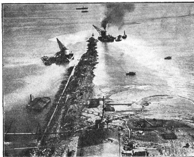
Travaux de remblayage de la grande digue.
