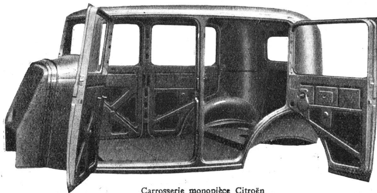
Carrosserie monopièce Citroën
