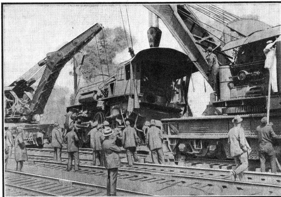
Deux puissantes grues soulèvent une locomotive dérailée, pour la reposer sur les rails.
