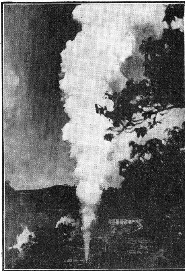
Vue d'un Soffiono de la vallée de Larderello. La vapeur s'en échappe avec force en un jet de plusieurs dizaines de mètres de haut.
