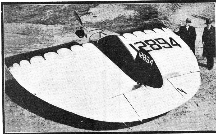
L'avion sans queue Arup «S-35» sans ailerons extrêmes, dont nous donnons la description. Cette photo nous a été confiée par la revue d'aviation « Les Ailes ».
