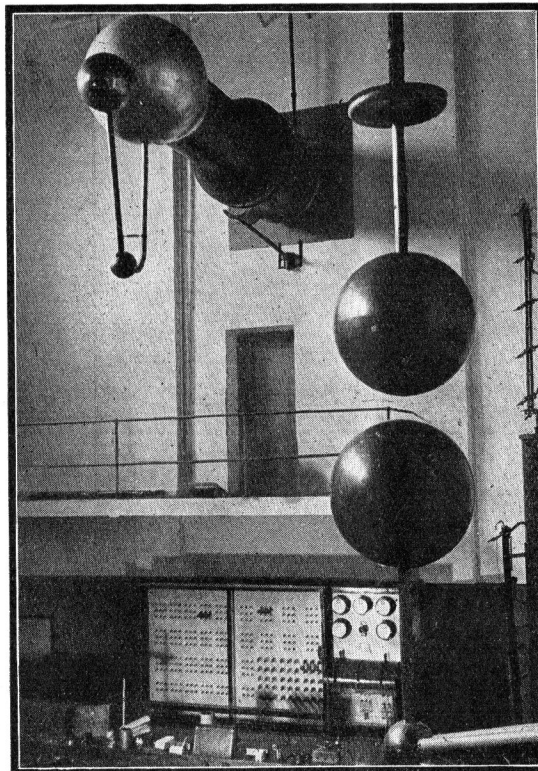
En haut : arc électrique entretenu, par courant alternatif, sous la tension de 1 million de volts. En bas : installations du laboratoire allemand de l'« A.E.G. » pour la production des étincelles de choc à haute tension.
