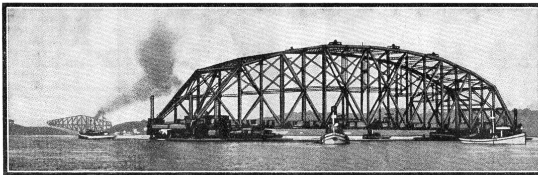
La portée centrale reposant sur les pontons, pendant son transport au centre du pont. On aperçoit, au fond, les deux cantilevers prêts à recevoir cette portée.
