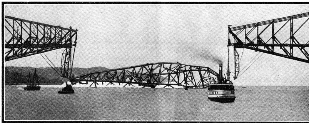
L'effondrement de la portée centrale, à 10 h. 50, le 11 Septembre 1916.
