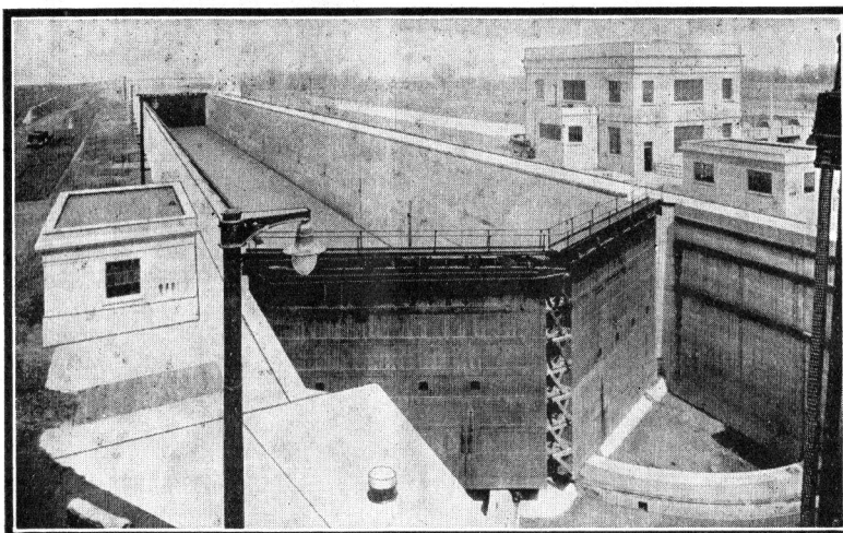
Vue d'une des sept écluses géantes du Canal de Welland qui relie le lac Ontario au lac Erié (Amérique du Nord). Chacune de ces écluses mesure 260 mètres de long sur 25 mètres de large, et fournit une élévation de 14 mètres.
