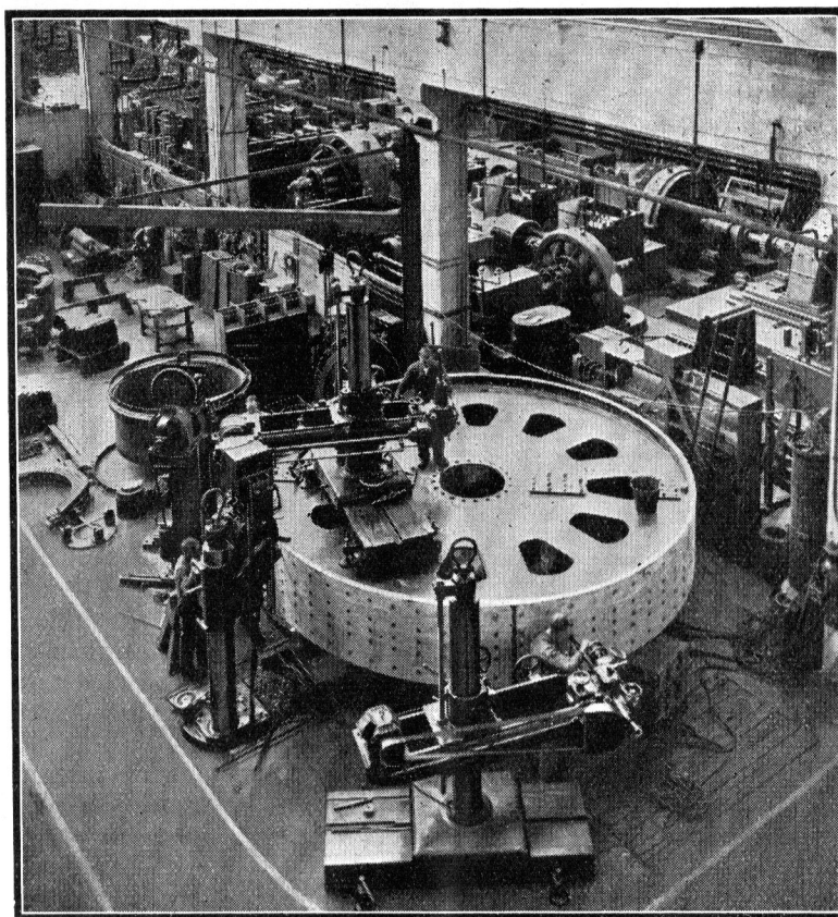
Percement de trous dans le bâti du rotor du plus grand moteur synchrone du monde, décrit dans cet article. Ce cliché nous a été gracieusement prêté par la British Thomson-Houston Company Ltd.
