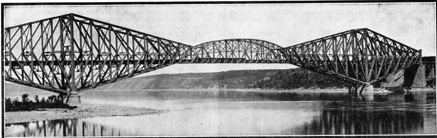
Vue générale du Pont de Québec.
