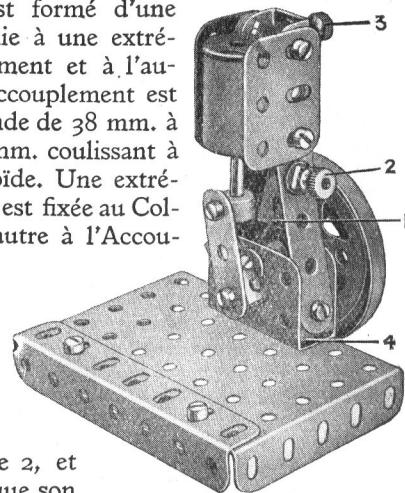
Fig. 5. Moteur électrique.
