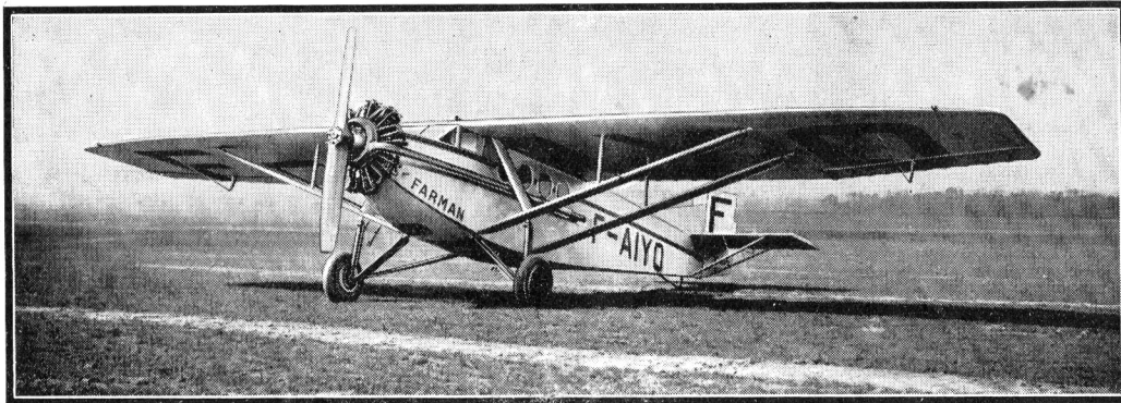
Vue du monoplan à ailes surélevées Farman « F-190 », muni d'un moteur de 300 CV. C'est avec un appareil de ce type que le pilote Génin a battu dernièrement le record de vitesse entre Marseille et Madagascar en accomplissant ce vol en 3 jours 13 heures 18 minutes. Photographie des Avions Farman .
