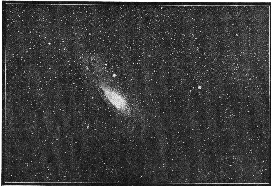
Vue de la grande nébuleuse d'Andromède, une des plus rapprochées de notre monde solaire et dont nous sépare une distance d'environ un million d'années-lumière. Les nébuleuses sont, on le sait, des agglomérations d'étoiles semblables à la Voie Lactée, dont fait partie notre soleil avec les planètes qui gravitent autour de lui.
