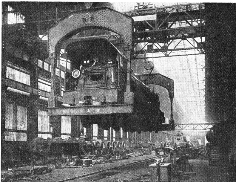
Une locomotive Pacific soulevée par deux ponts roulants de 60 tonnes dans un hall des Ateliers de Sotteville des Chemins de fer de l'Etat. Cliché de la Revue Pittoresque des Chemins de Fer .
