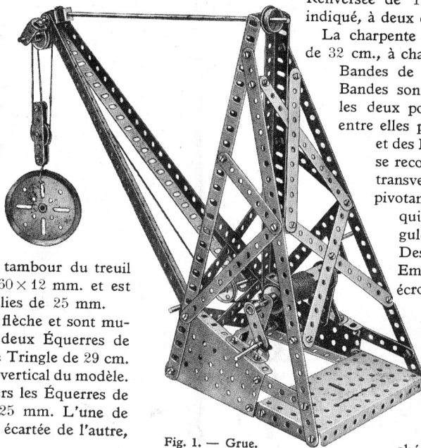
Fig. 1. — Grue.
