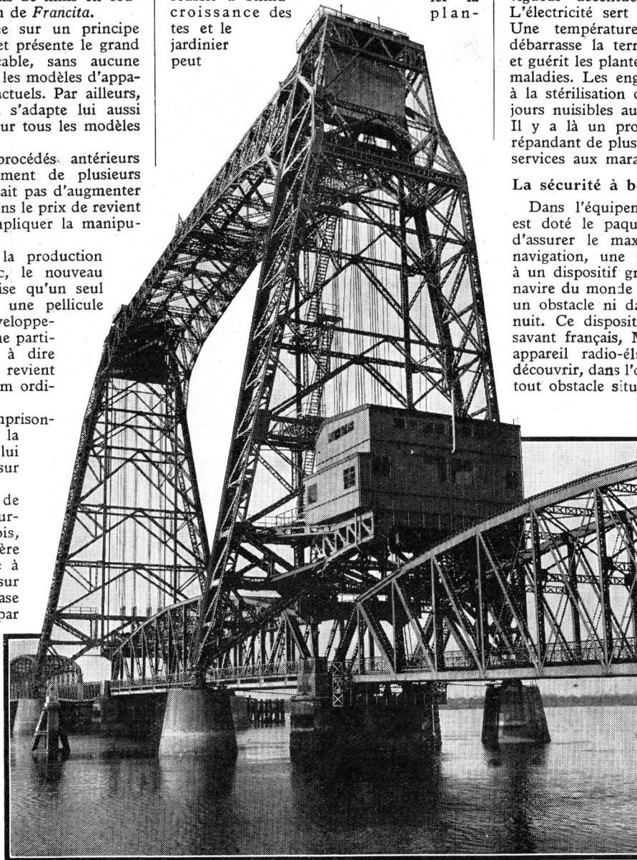
Vue impressionnante du pont-ascenseur de Barendrecht, en Hollande, qui est une des plus grandes constructions de ce type au monde.
