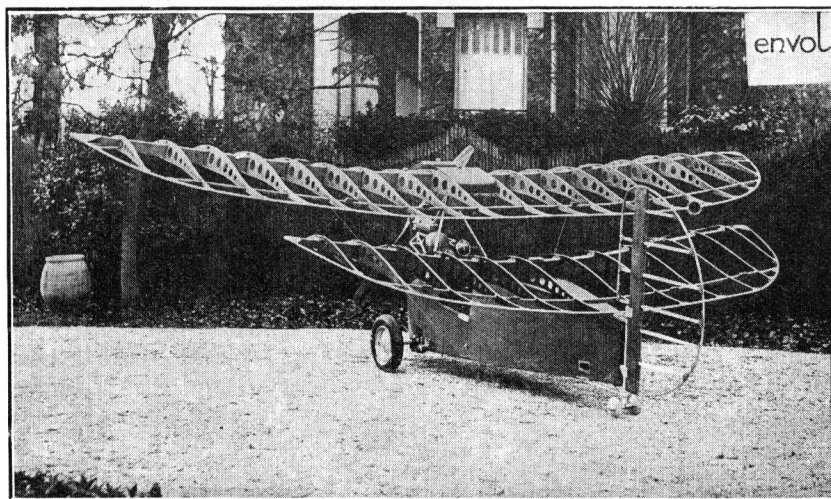
Ci-dessus : squelette d'un "Pou-du-Ciel". En haut et ci-contre : deux "Poux-du-Ciel", photographiés sur leurs terrains d'aviation. Ces clichés nous ont été confiés par la revue "Envol", organe du Réseau des Amateurs de l'Air.
