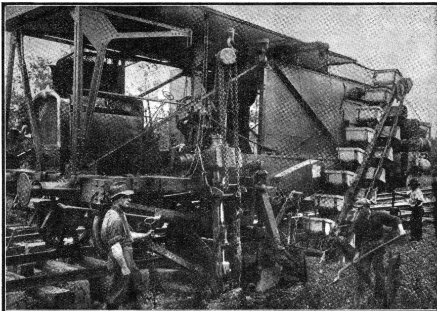
La machine Scheuchzer ; vue d'ensemble.
