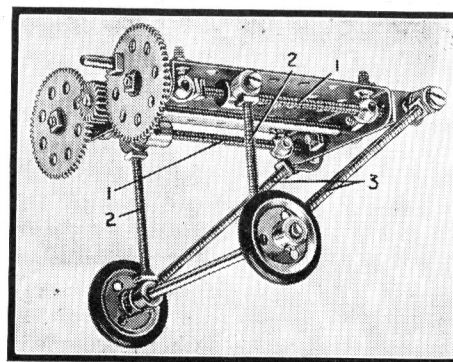
Fig. 2. Train d'atterrissage escamotable en vol.
