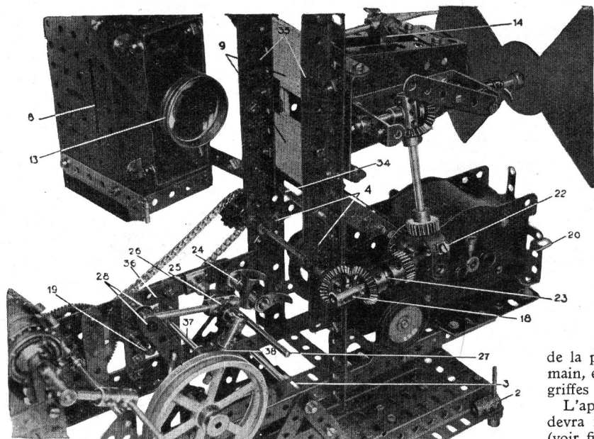
Fig. 2. — Vue de la partie centrale du modèle.
