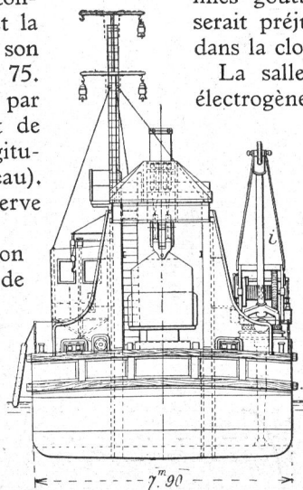
Fig. 2. Vue en bout du ponton-grue.
