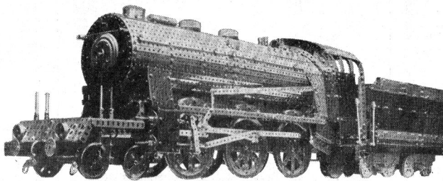
Ce superbe modèle de locomotive « Pacific » 4-6-2, mesurant 1 m. 50 de long et pesant plus de 20 kg, a été construit par M. G. Boschet, de Lyon, gagnant du 14 e prix à notre dernier Grand Concours National (Section C).
