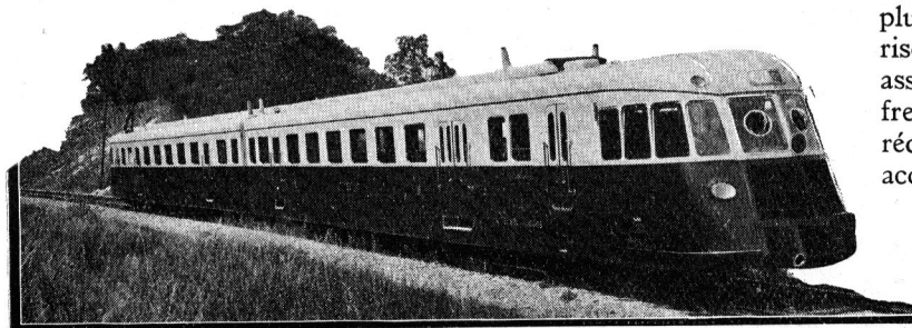
Fig. 9. — Autorail Renault type A.B.V. des Chemins de fer de l'Est.
