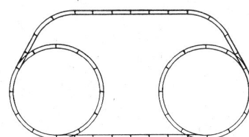
Rayon de 61 cm. (ci-dessus) 24 Rails courbes (A2) 14 Rails droits (B1) 2 Aiguilles droites (PR2) 2 Aiguilles gauches (PL2) Dim. : 3 m 65 × 1 m 50
