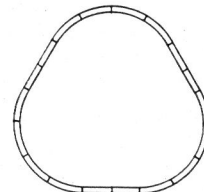
Rayon de 61 cm. (ci-dessus) 12 Rails courbes (A2) 6 Rails droits (B1) Dim. : 1 m 85 × 1 m 85
