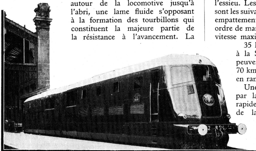
Fig. 4. — Locomotive Diesel électrique à grande vitesse de 4.000 chevaux du P.-L.-M.
