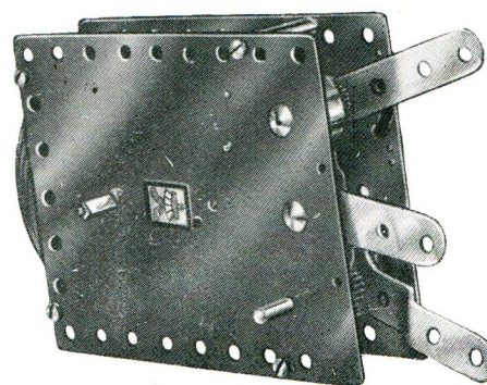
MOTORE AD OROLOGERIA Tipo G Con 2 velocità retromarcia e freno
